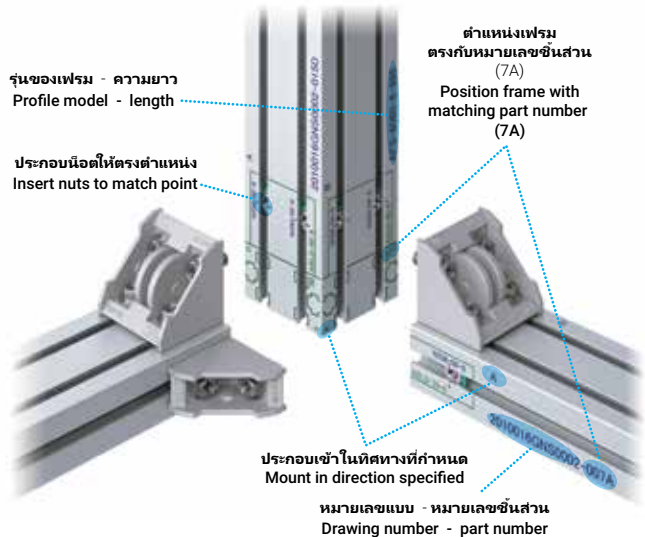
ส่วนประกอบ (ที่ Mark แล้ว) + อลูมิเนียมเฟรมพร้อมน็อต + แบบสำหรับการประกอบ Components (Marked) + Aluminum frame with the nut + Assembly drawing
